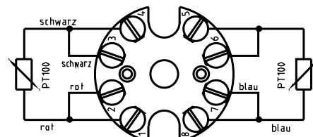
2 PT100- 4 Leiterschaltung
